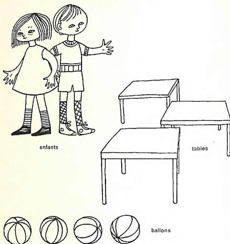
Fig. 12 NON-ÉQUIVALENCE D'ENSEMBLES
