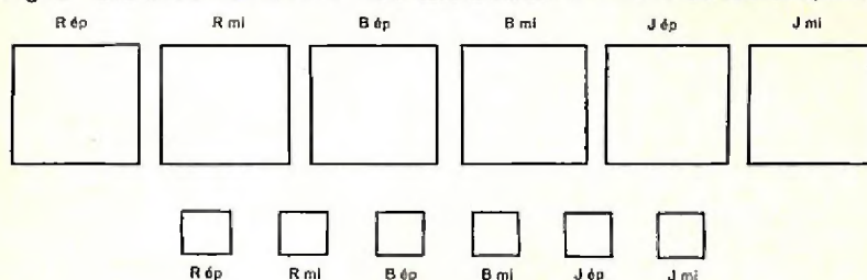
Fig. 3 NOTRE UNIVERS EST LA BOÎTE DE BLOCS LOGIQUES
