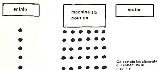
Fig. 24 MACHINES D'ENSEMBLES D'ENSEMBLES. EXERCICE COMPRENANT UN « PATRON »
