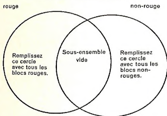
Fig. 8 ENSEMBLE COMPLÉMENTAIRE
