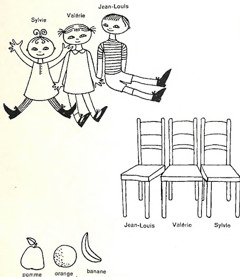
Fig. 11 ENSEMBLES ÉQUIVALENTS
