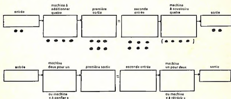
Fig. 26 MACHINES « INVERSES » — MACHINES QUI NE FONT RIEN
