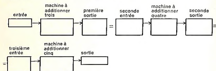
Fig. 28 COMMUTATIVITÉ (suite)
