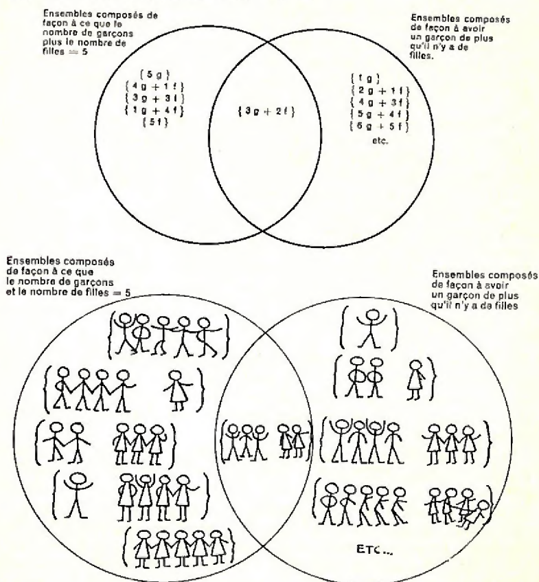
Fig. 18 ENSEMBLES D'ENSEMBLES
