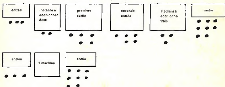
Fig. 23 MACHINES ÉQUIVALENTES : UNE MACHINE FAIT LE TRAVAIL DE DEUX MACHINES
