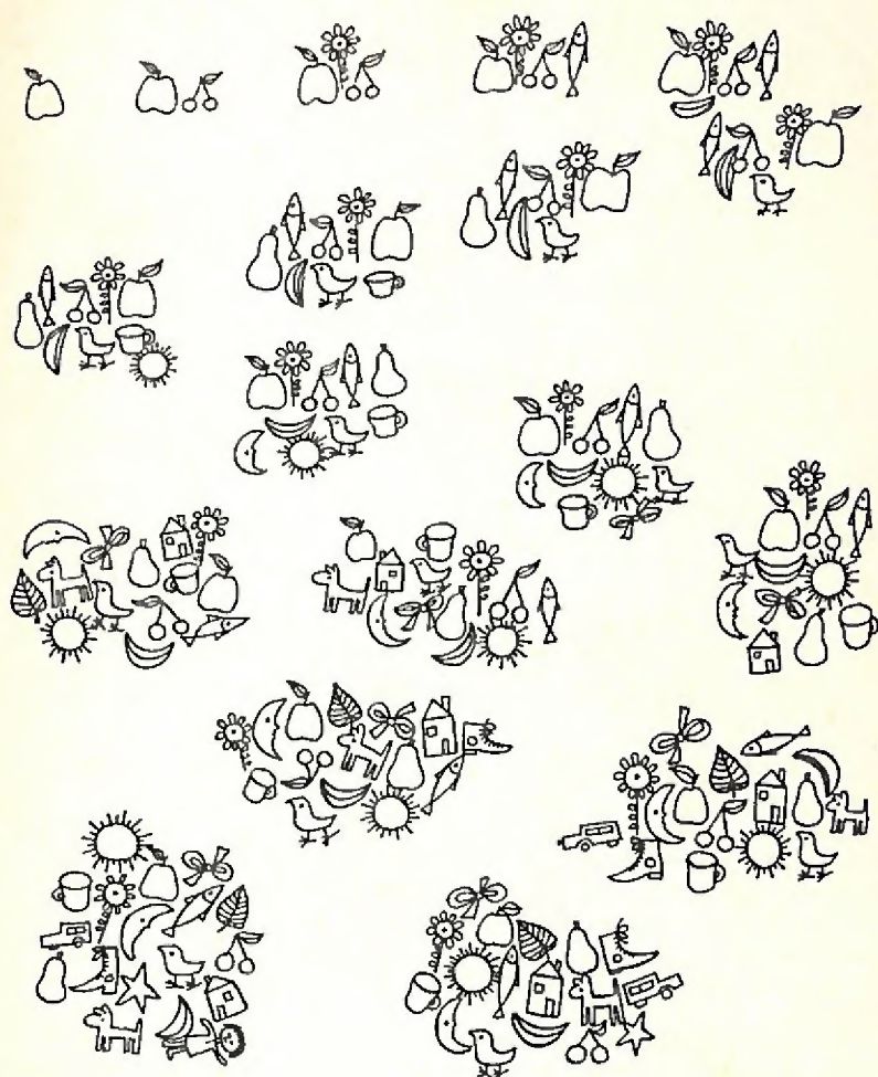
Fig. 13 NON-ÉQUIVALENCE DES TAS QUI AUGMENTENT
